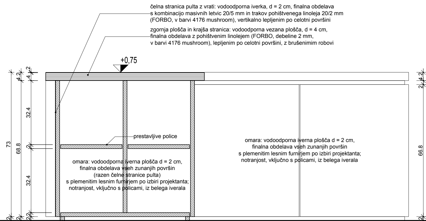
PREREZ 5
