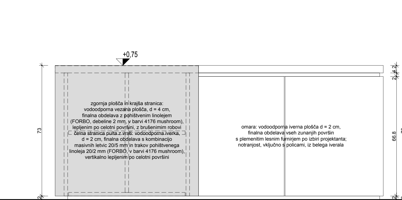
POGLED 6
