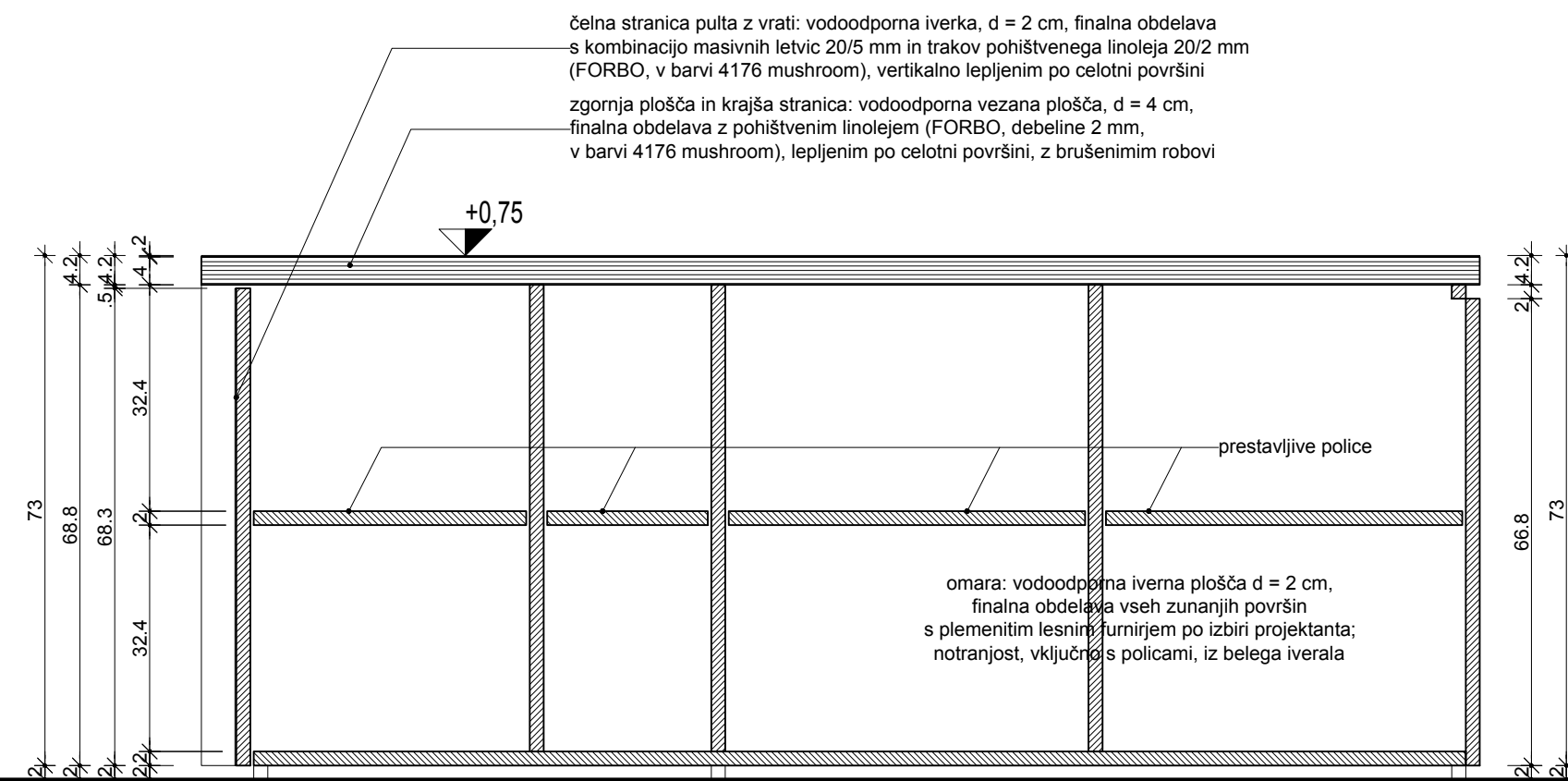
PREREZ 3
