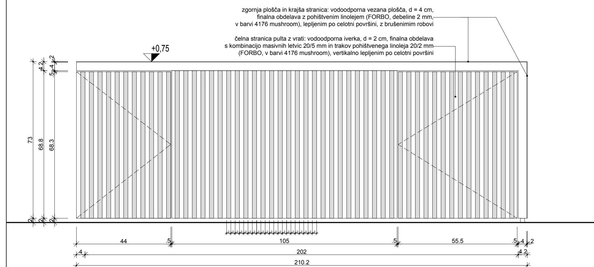
POGLED 1
