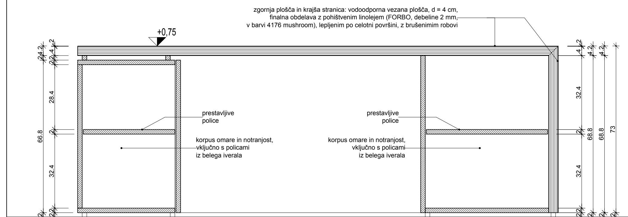
PREREZ 2
