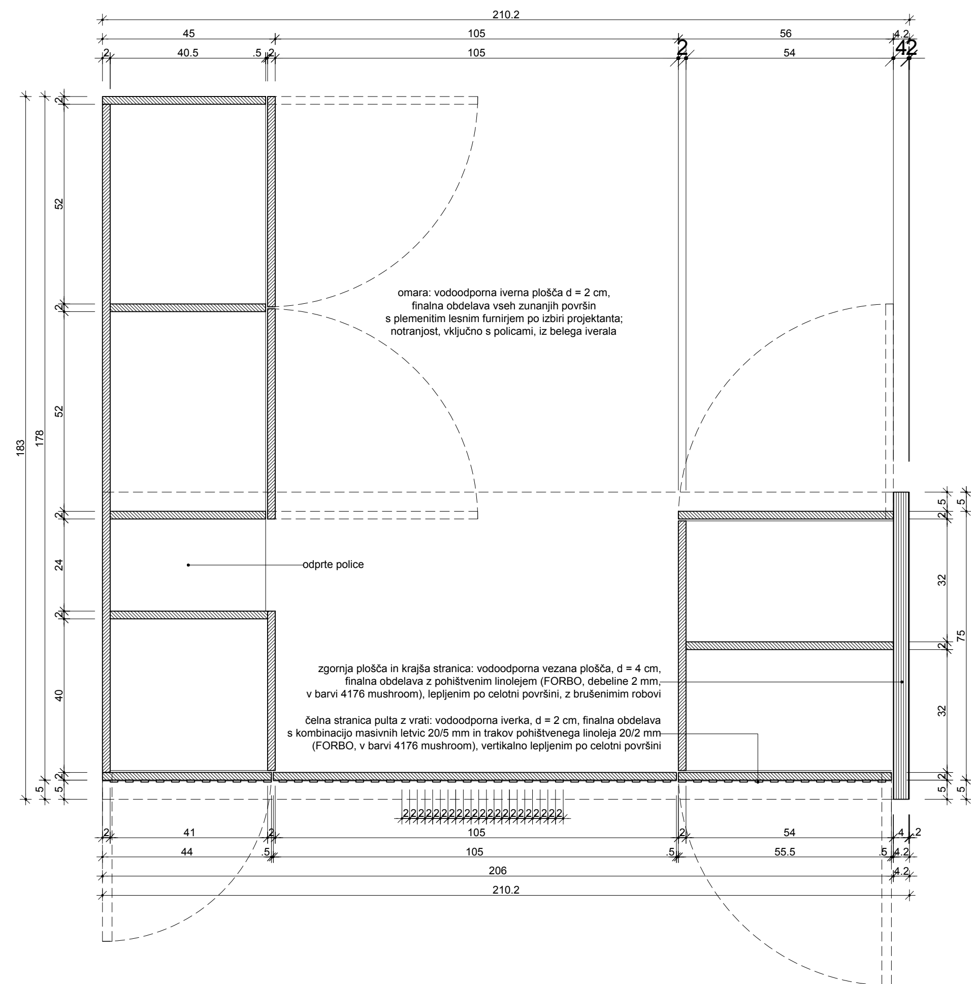
PREREZ 4
