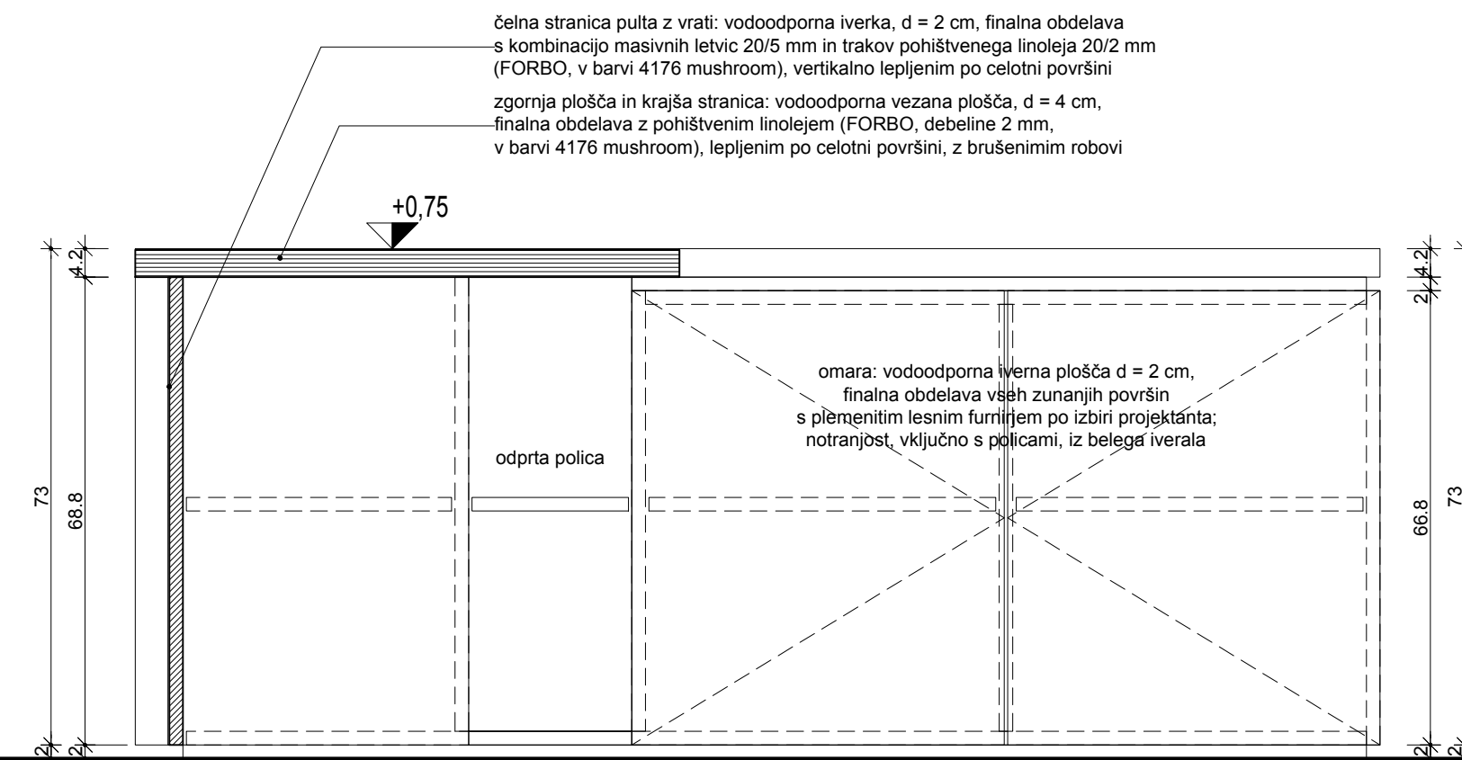
PREREZ 4
